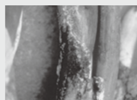
黒腐菌核病
