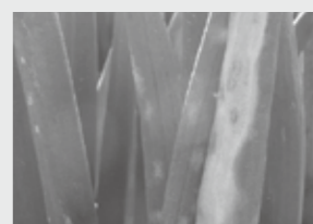
さび病
